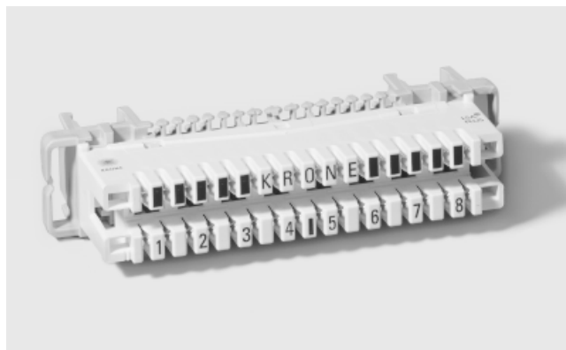
LSA PROFIL disconnection module 2/8
