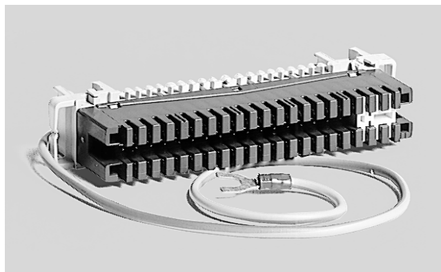
LSA PROFIL earth module 2/34
